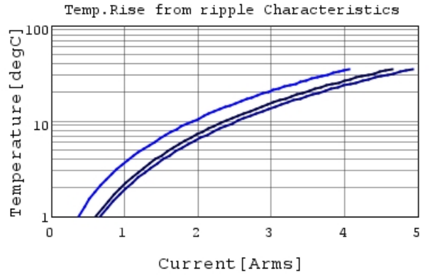
GCJ31CR71A226KE01 Temp.rise — 80kHz
