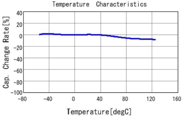
■ GCJ188R71H472KA01 C-Temp. capchange, DCO. 0V, AC1. 0Vrm
