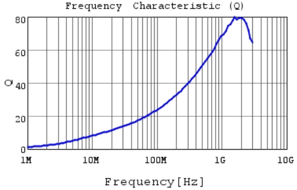
LQW15AN18NJ80 Q
