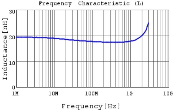
LQW15AN18NJ80 L
