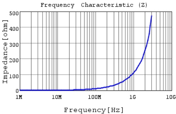
LQW15AN18NJ80 |Z|
