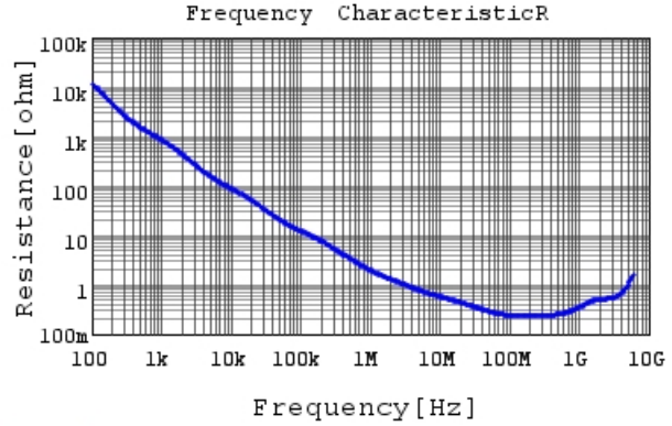
GRM033B11E102KA01 R DCOV, 20degC
