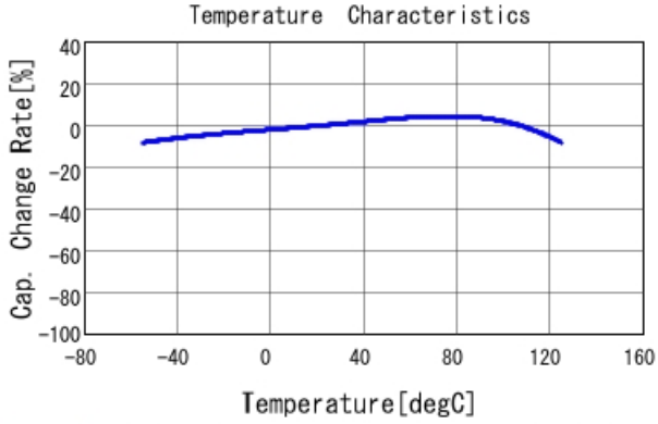
GCM21BR71A106KE22 C-Temp. capchange, DCO. 0V, ACO. 5
