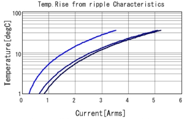
GCM21BR71A106KE22 Temp. rise — 80kHz — 400kHz
