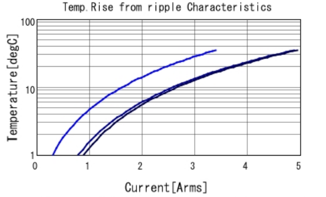
GRM319B31C106KE15 Temp. rise — 80kHz — 400kHz
