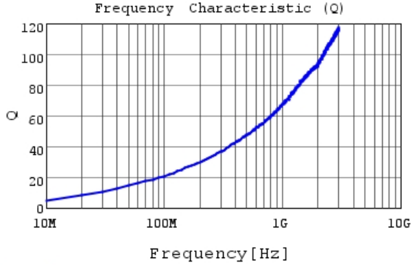
LQW15AN6N2B00 Q
