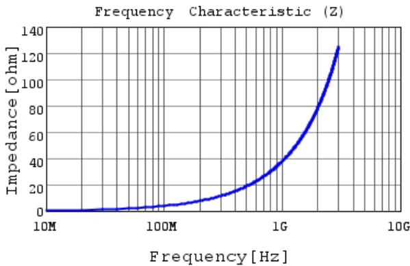
LQW15AN6N2B00 |Z|
