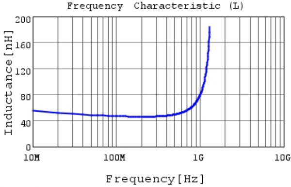
LQG15HH47NH02 L
