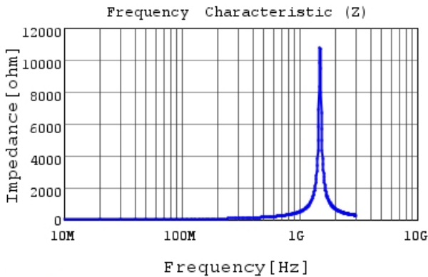
LQG15HH47NH02 |Z|
