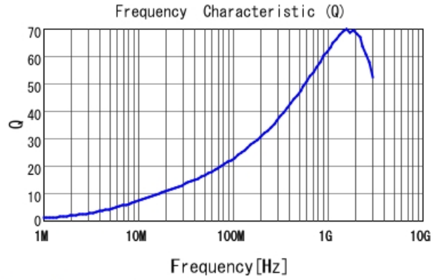
LQW15AN23NJ80 Q
