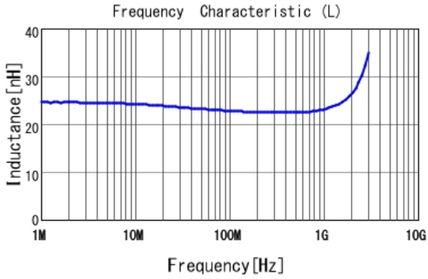
LQW15AN23NJ80 L
