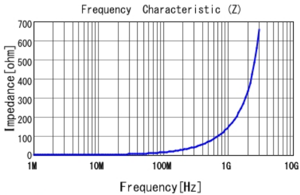
LQW15AN23NJ80 |Z|
