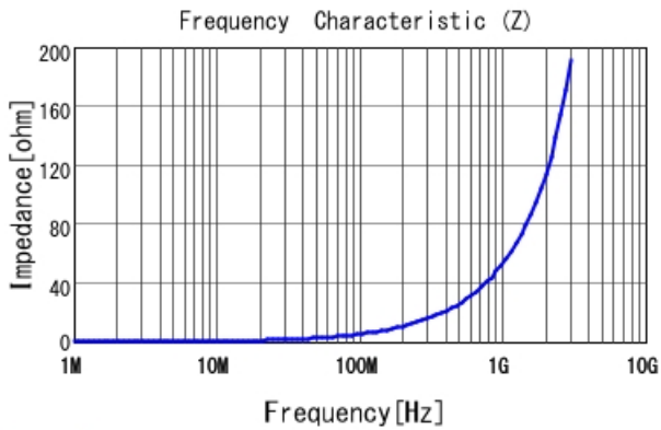
LQW15AN8N5G80 |Z|
