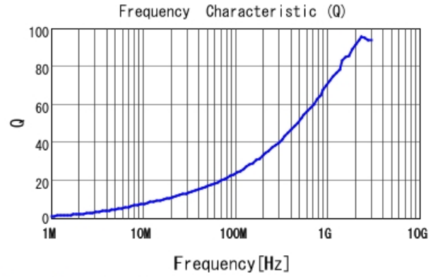
LQW15AN8N5G80 Q
