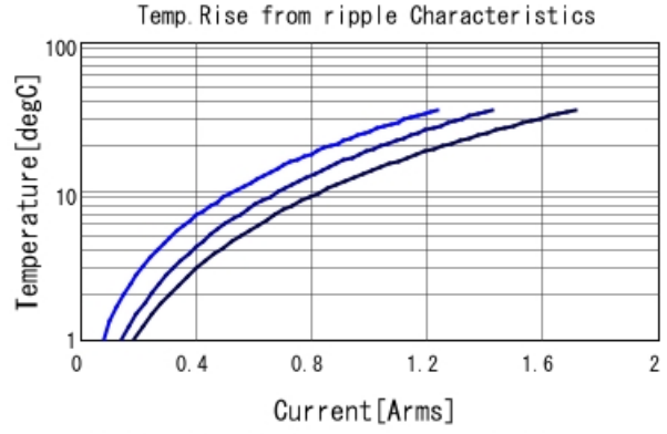
GRM155R6YA224KE01 Temp. rise — 300kHz — 600I
