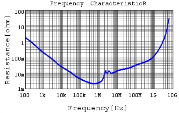
GRM32ER71E226ME15 R DCOV, 25degC
