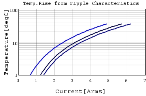
GRM32ER71E226ME15 Temp.rise — 80kHz —
