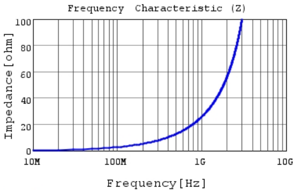
LQG15HZ4N3C02 |Z|
