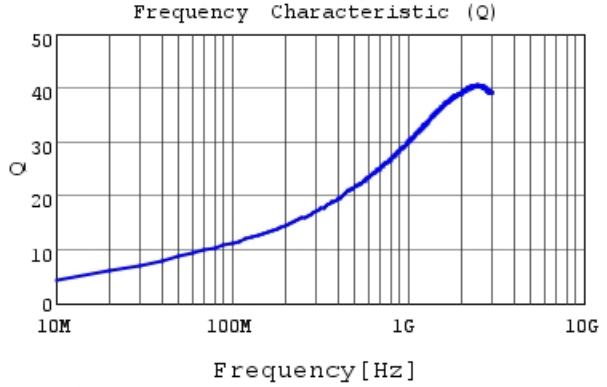
LQG15HZ4N3C02 Q
