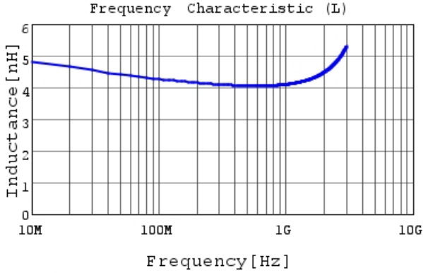
LQG15HZ4N3C02 L
