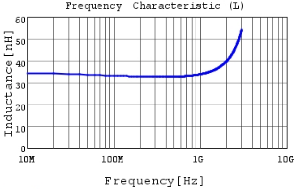
LQW15AN33NJ00 L
