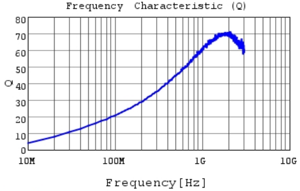
LQW15AN33NJ00 Q
