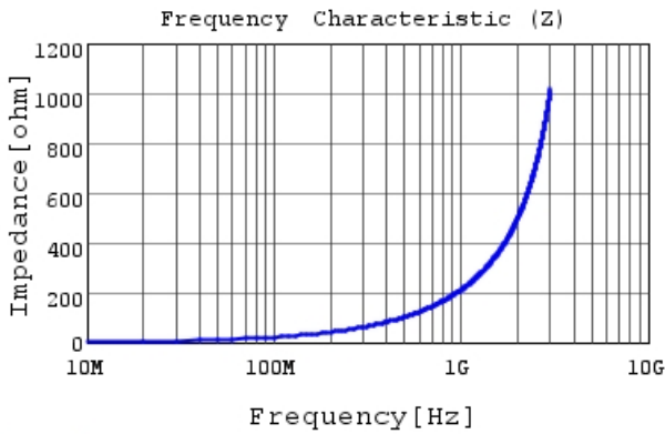
LQW15AN33NJ00 |Z|
