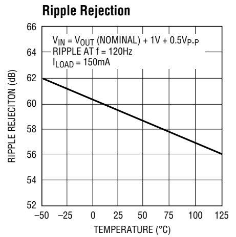
LT1521 • TPC30
