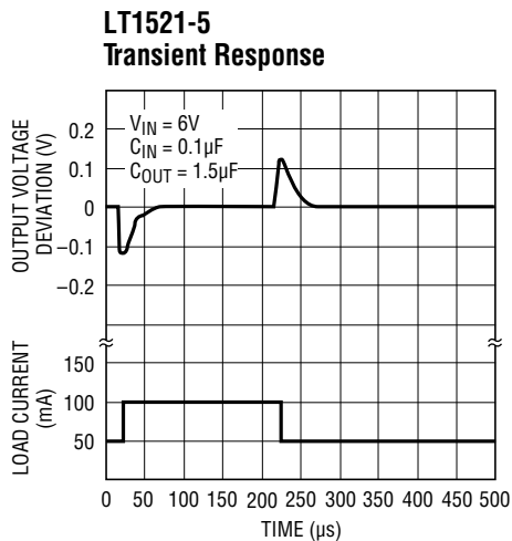
LT1521 • TPC33
