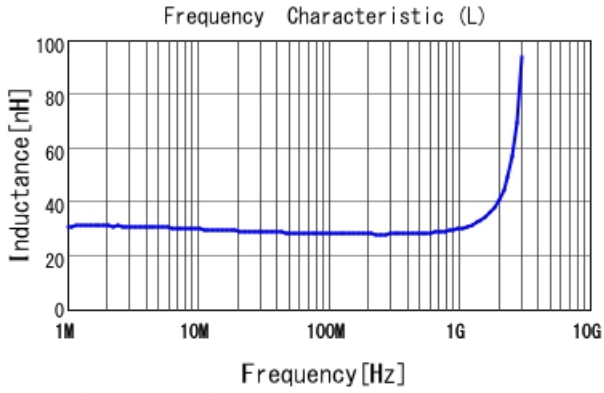
LQW18AN28NJ8Z L
