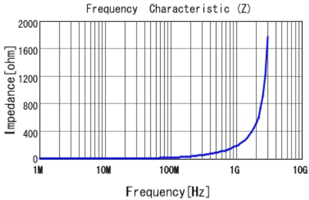
LQW18AN28NJ8Z |Z|
