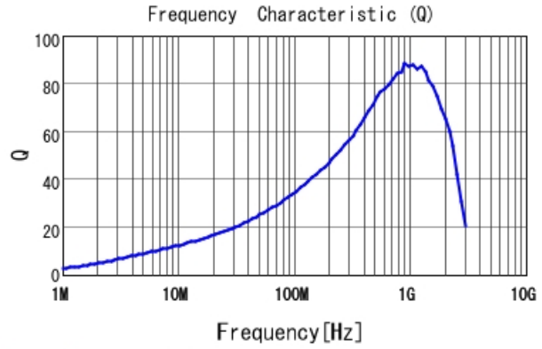
LQW18AN28NJ8Z Q
