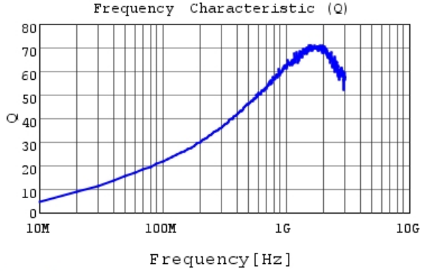
LQW15AN39NG00 Q
