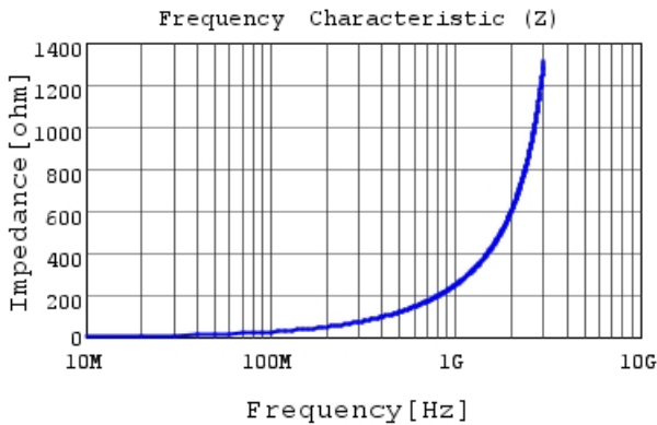
LQW15AN39NG00 |Z|
