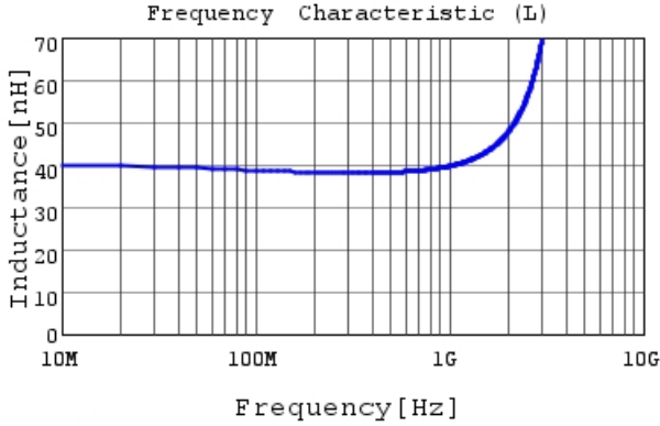
LQW15AN39NG00 L
