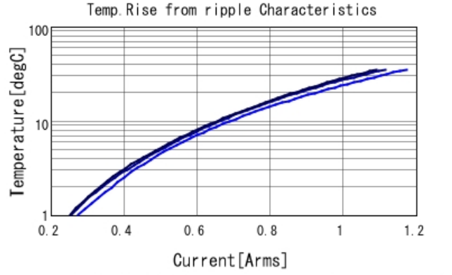
GQM2195C2E120JB12 Temp. rise — 500MHz — 700
