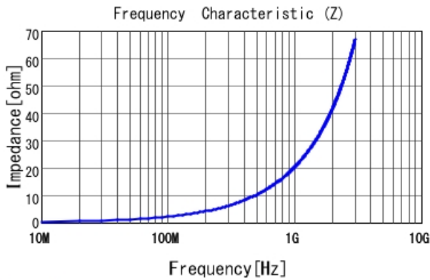
LQP03TN3N2BZ2 |Z|
