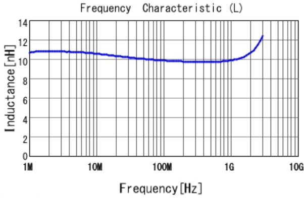
LQW15AN9N7J8Z L
