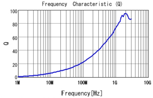
LQW15AN9N7J8Z Q
