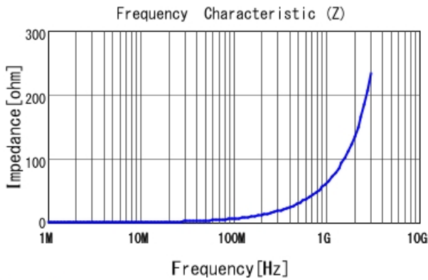
LQW15AN9N7J8Z |Z|
