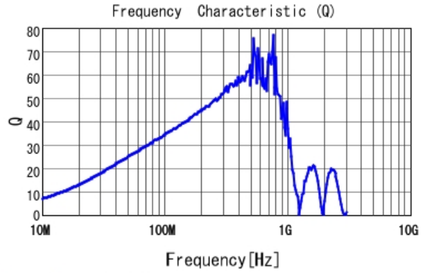
LQW18ANR30G8Z Q
