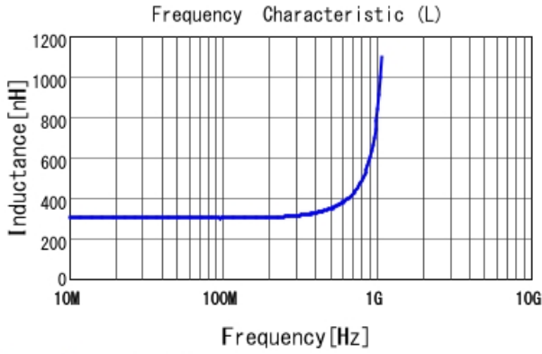
LQW18ANR30G8Z L
