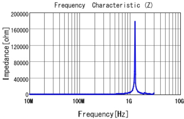
LQW18ANR30G8Z |Z|
