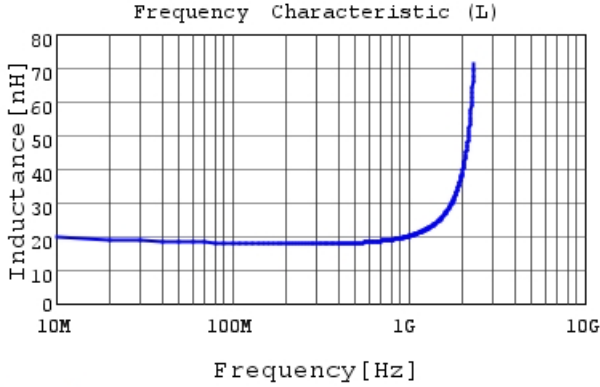
LQG18HN18NJ00 L
