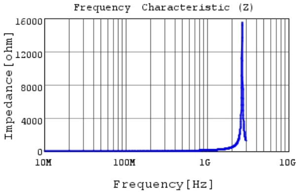
LQG18HN18NJ00 |Z|
