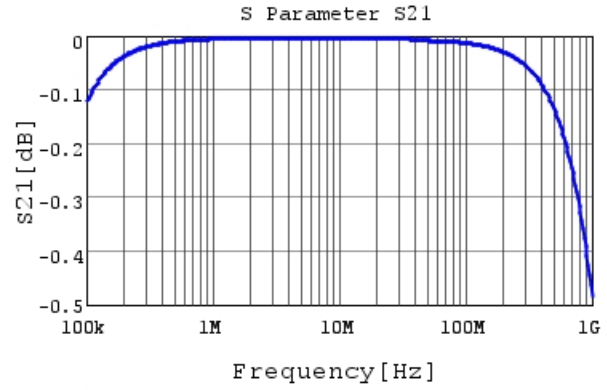
RDER71H104K0P1H03B S21 DC0V, 25degC
