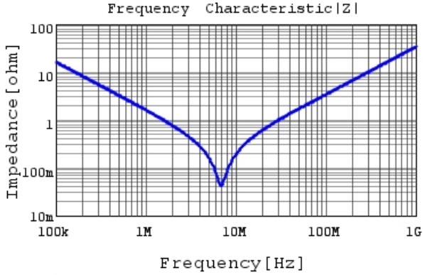
RDER71H104K0P1H03B |Z| DC0V, 25degC
