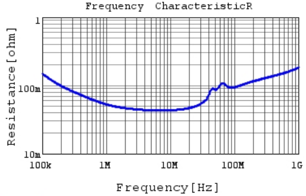
RDER71H104K0P1H03B R DC0V, 25degC
