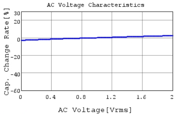
RDER71H104K0P1H03B C-AC Voltage capchange, I
