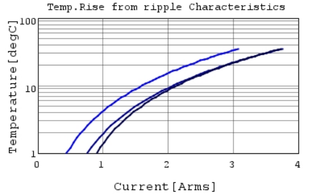
GRM155R61A475MEAA Temp.rise — 100kHz —
