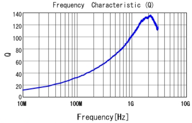
LQW18AN12NG1Z Q
