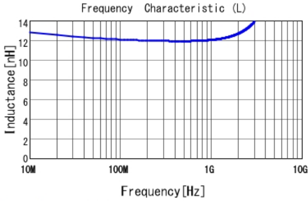
LQW18AN12NG1Z L
