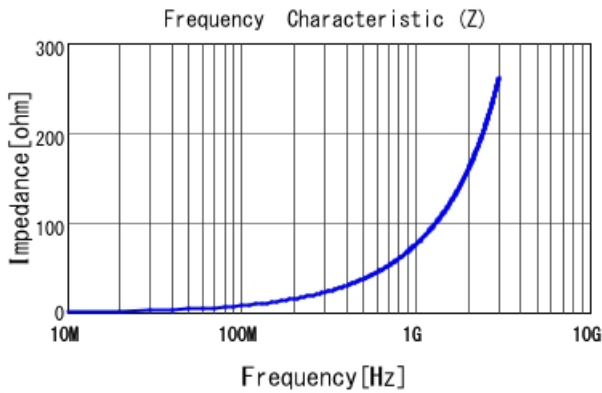
LQW18AN12NG1Z |Z|
