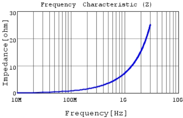
LQG15HS1N2B02 |Z|
