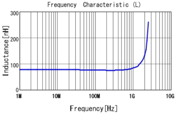
LQW15AN75NJ8Z L
