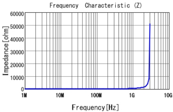
LQW15AN75NJ8Z |Z|
