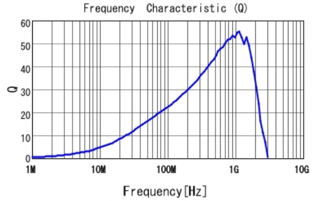
LQW15AN75NJ8Z Q
