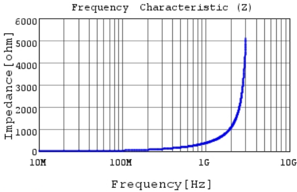
LQW15AN56NG00 |Z|
