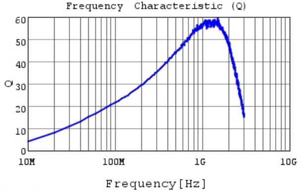
LQW15AN56NG00 Q
