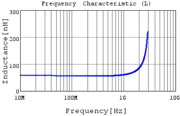
LQW15AN56NG00 L
