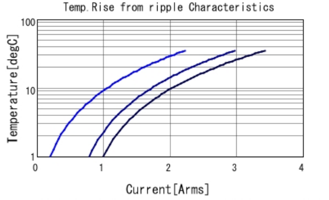
GRM155R61A105KE15 Temp. rise — 100kHz — 500
