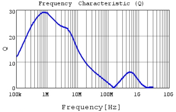
LQH2HPZR68MGR Q
