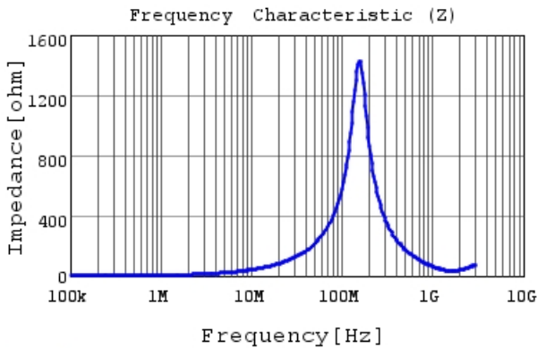
LQH2HPZR68MGR |Z|
