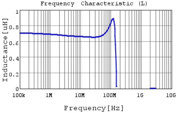
LQH2HPZR68MGR L
