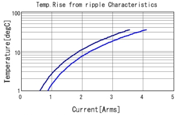
GRM21BR71H105KA12 Temp. rise — 500kHz — 1MHz
