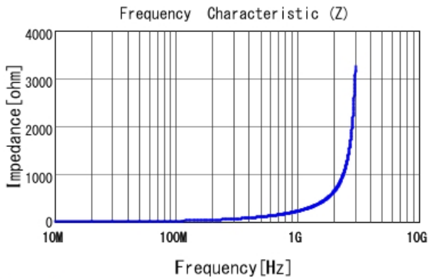
LQW18AN33NJ0Z |Z|
