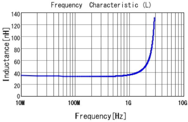
LQW18AN33NJ0Z L
