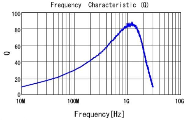
LQW18AN33NJ0Z Q
