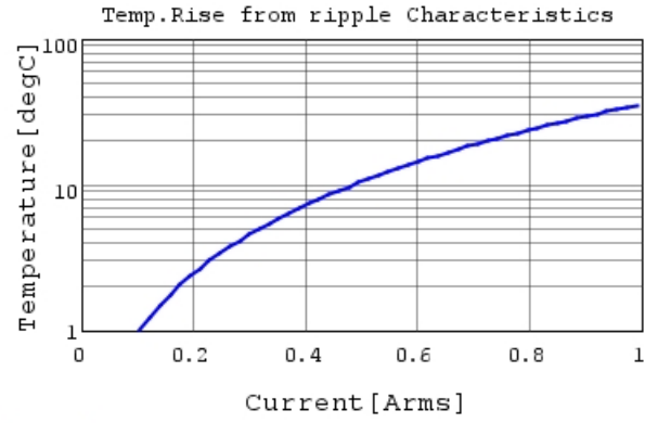
GRM033R60J104KE19 Temp.rise 800kHz
