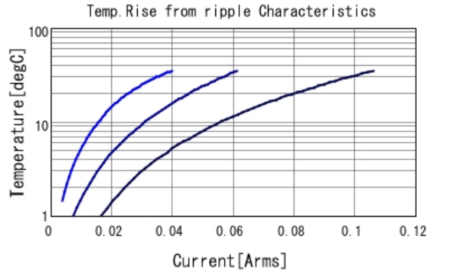
GCJ21AR72E102KXJ1 Temp. rise — 30kHz — 100kHz
