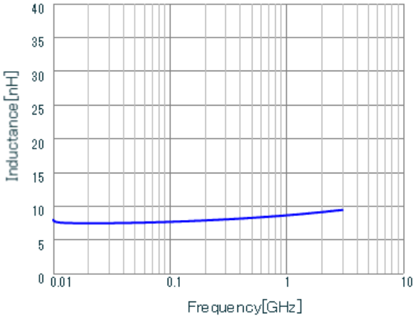
LQW18AN7N5C8Z L.
