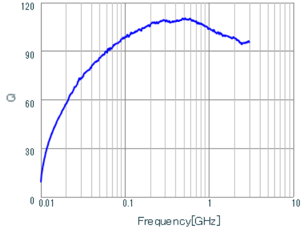
LQW18AN7N5C8Z Q.
