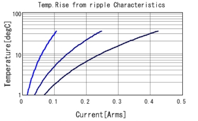
GRM31CR73A103KW03 Temp. rise — 30kHz — 100kHz
