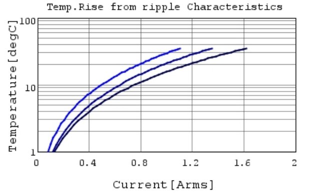
GRT155R61E224KE01 Temp.rise — 300kHz —
