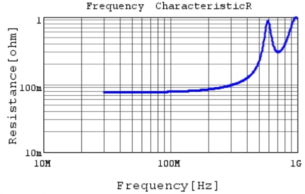
RDE5C1H561J0M1H03A R DCOV,25degC
