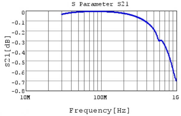
RDE5C1H561J0M1H03A S21 DCOV, 25degC
