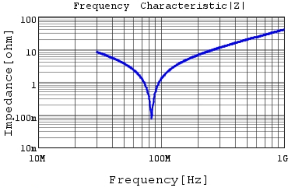
RDE5C1H561J0M1H03A |Z| DCOV,25degC
