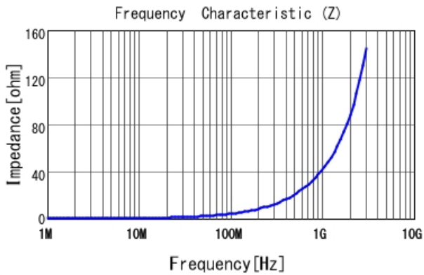
LQW15AN6N6G8Z |Z|
