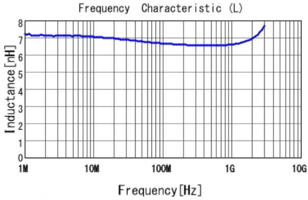
LQW15AN6N6G8Z L
