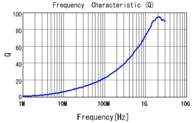
LQW15AN6N6G8Z Q
