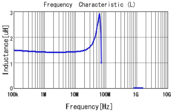
1267AY-1R5N L
