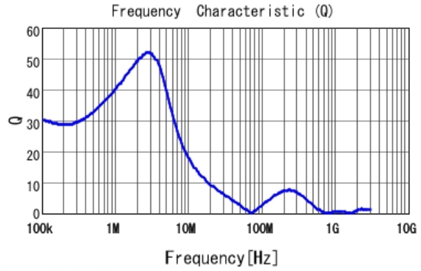
1267AY-1R5N Q
