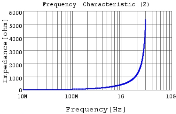
LQW15AN62NJ00 |Z|
