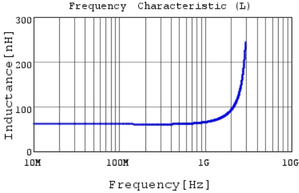
LQW15AN62NJ00 L
