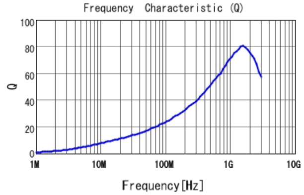
LQW15AN19NG80 Q
