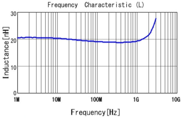
LQW15AN19NG80 L
