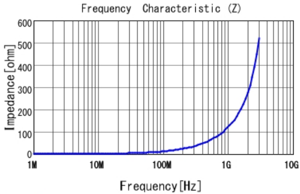
LQW15AN19NG80 |Z|
