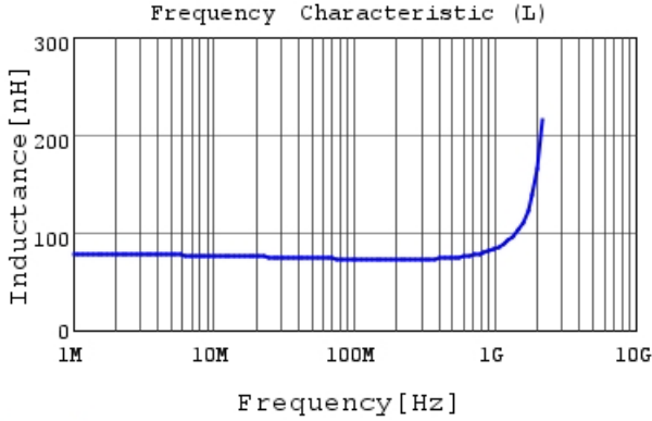
LQW18AN73NJ8Z L
