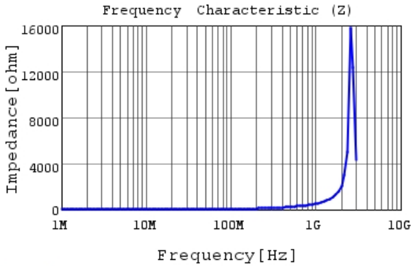
LQW18AN73NJ8Z |Z|
