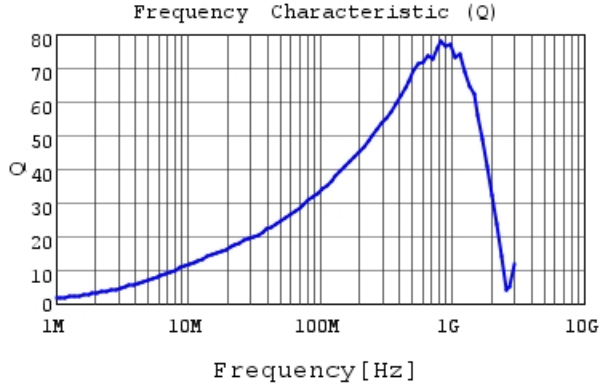
LQW18AN73NJ8Z Q
