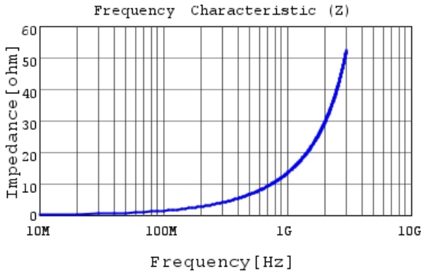
LQG15HH2N2S02 |Z|
