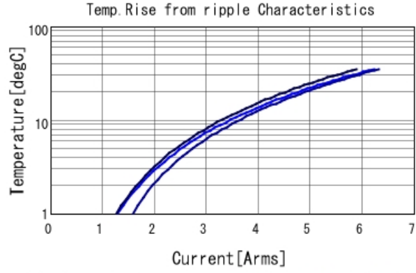
GRM21BB30G476ME15 Temp. rise ■ 60kHz ■ 300kHz ■ 600kHz
