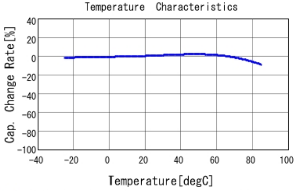
■ GRM21BB30G476ME15 C-Temp. capchange, DCO. 0V, ACO. 2Vrm
