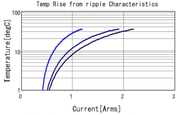
GRM188R61E474KA12 Temp. rise — 200kHz — 500
