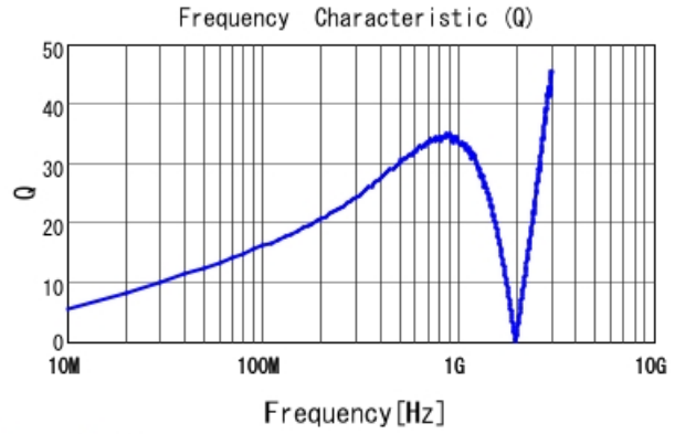
LQG15WZ47NH02 Q
