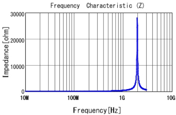
LQG15WZ47NH02 |Z|
