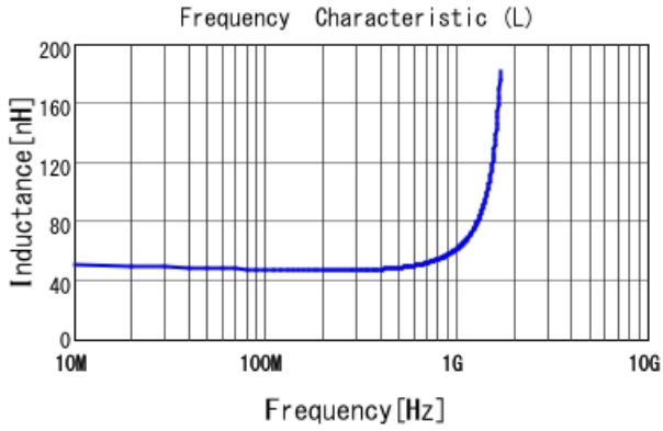
LQG15WZ47NH02 L
