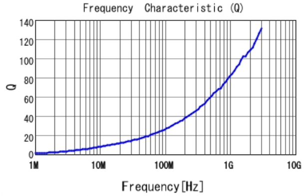
LQW15AN3N7G8Z Q
