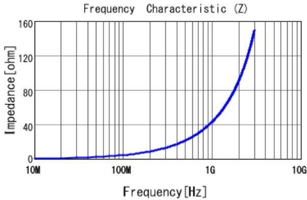
LQW15AN7N0G00 |Z|
