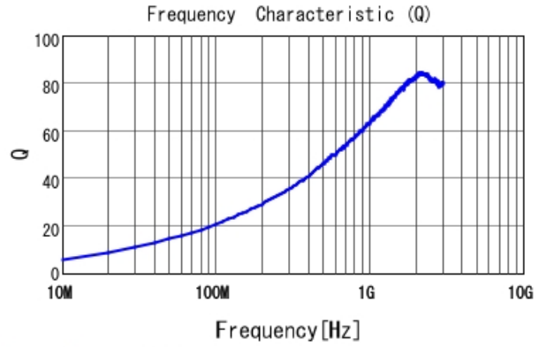
LQW15AN7N0G00 Q
