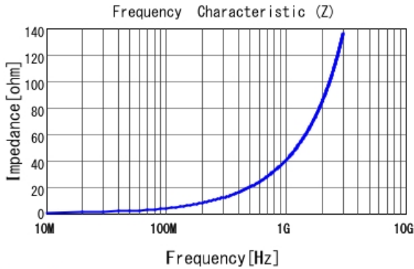
LQW15AN6N6B00 |Z|
