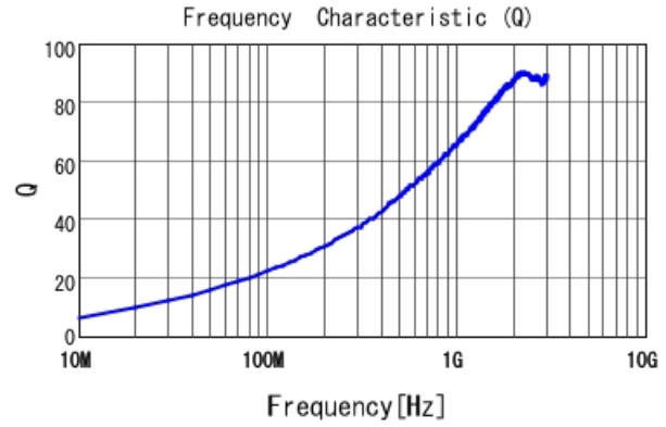
LQW15AN6N6B00 Q
