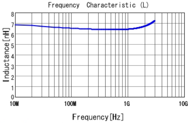
LQW15AN6N6B00 L
